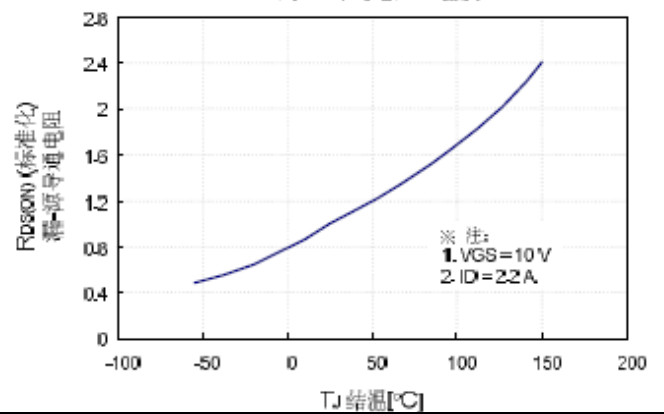
图8、导通电阻vs.温度
