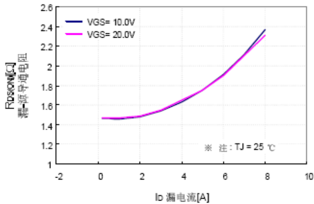
图3、导通电阻 vs. 漏电流和栅极电压
