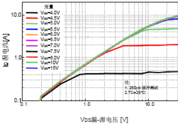
图1、导通电阻
