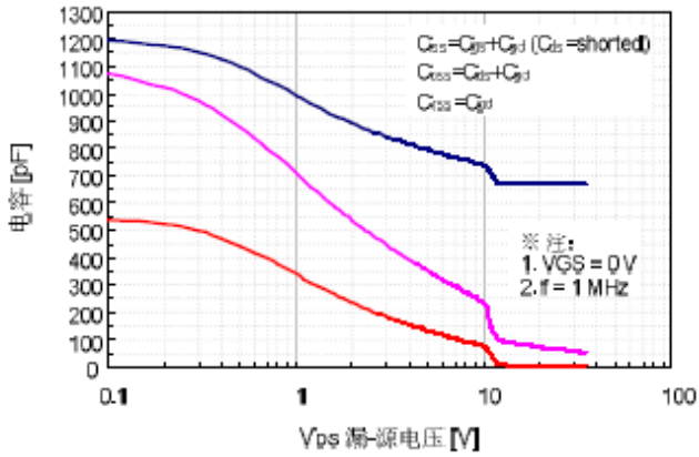
图5、电容特性
