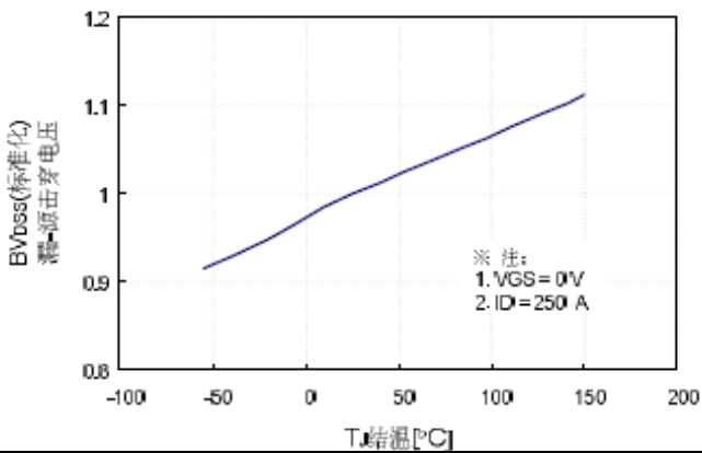
图7、击穿电压vs.温度
